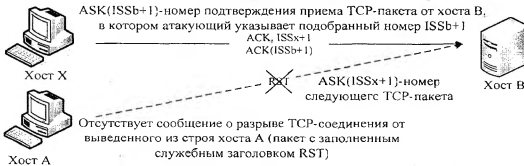
Рисунок 7. «Схема реализации угрозы «Подмена доверенного объекта сети»
