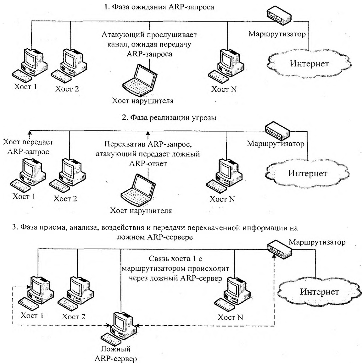
Рисунок 10. «Схема реализации угрозы «Внедрение ложного ARP-сервера»
